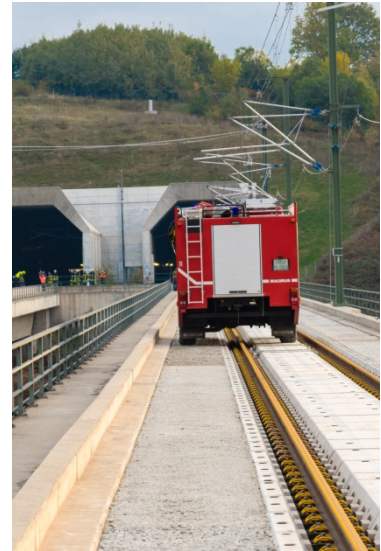
Abbildung 48: Befahrbares Gleis
